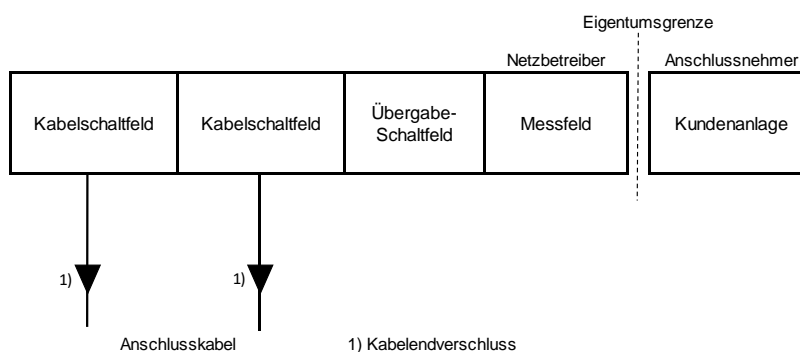
Prinzipdarstellung Mittelspannungsanschluss
