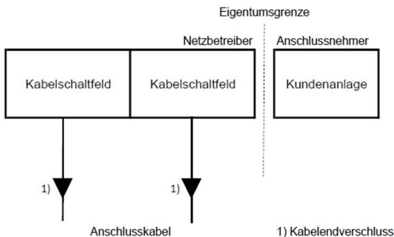
Prinzipdarstellung Mittelspannungsanschluss
