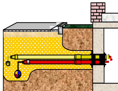
Abbildung 6: Mehrspartengebäudeeinführung für Gebäude mit Keller (2/4 Medien)
