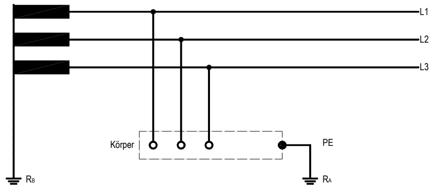
TT - System Dreileiternetz
