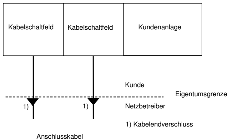
Prinzipdarstellung Mittelspannungsanschluss
