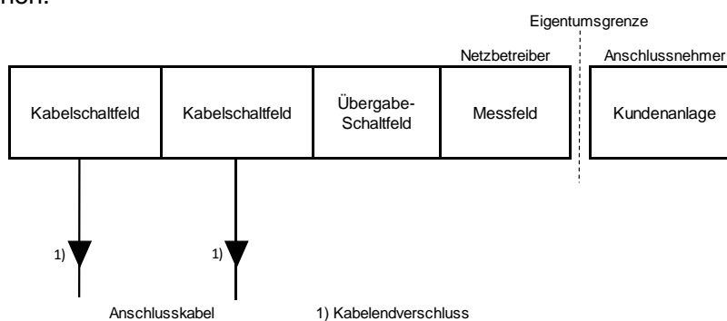
Prinzipdarstellung Mittelspannungsanschluss
