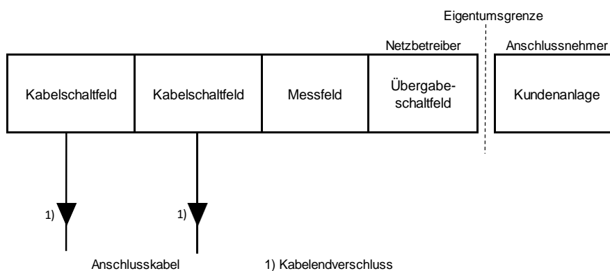
Prinzipdarstellung Mittelspannungsanschluss
