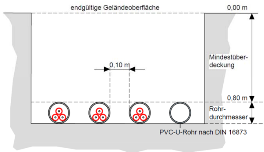
Abbildung 7-5 Mindestlegetiefe
